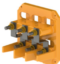
Figura 12 - Placa de bornes para carcaça 355A/B
