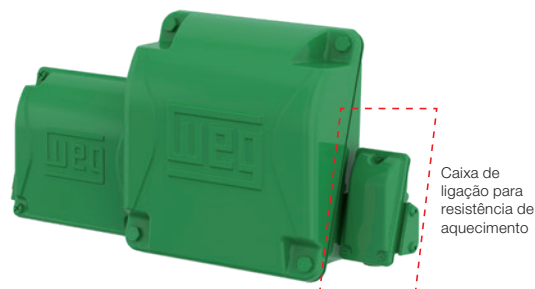
Figura 14 - Duas caixas de ligação de acessórios montadas junto à caixa de ligação principal.
